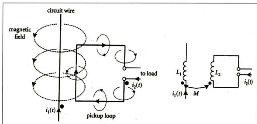
Bild 3: Faraday-Gesetz (Prinzip)
