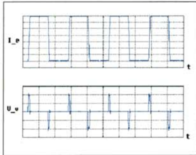
Bild 4: Beispiel Strom auf Emittor und induzierte Spannung auf dem Victim-Schaltkreis
