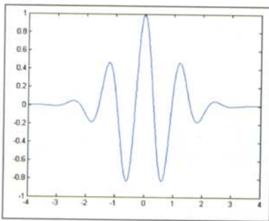
Bild 6: Beispiel eines Wavelets: Morlet Wavelet
